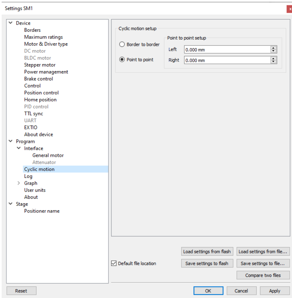
Рис. 5.36: Окно вкладки «Режим циклического движения»
