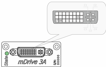
Рис. 4.8: Нумерация выводов в разъеме DVI-I, вид спереди
