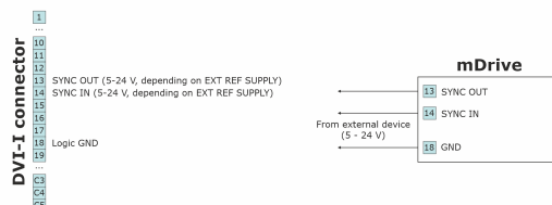
Рис. 4.40: Схема подключения к каналам синхронизации контроллера
