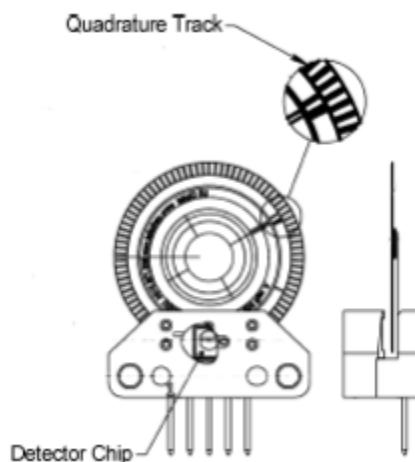
Рис. 4.20: Механика оптического квадратурного энкодера
