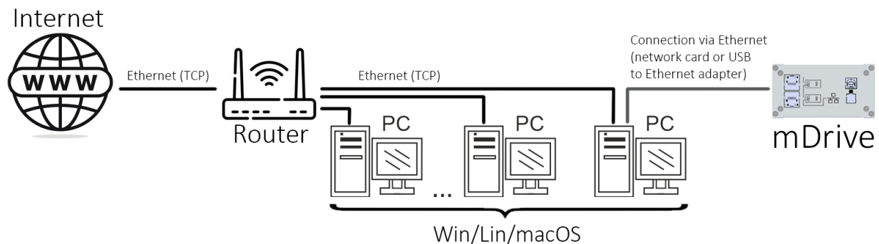
Рис. 7.4: На схеме показано, что, подключив контроллер к компьютеру с помощью кабеля Ethernet или USB - Ethernet адаптера, вы можете найти его в сети и работать с ним. Все компьютеры в сети могут иметь доступ к этому контроллеру
