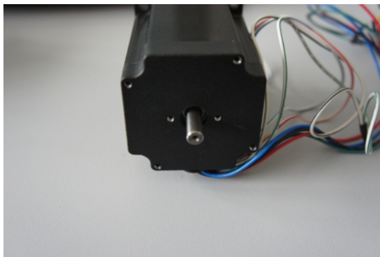
Рис. 3.8: Мотор без энкодера. Обратите внимание на 2 отверстия M2.5 к которым обычно крепится энкодер
