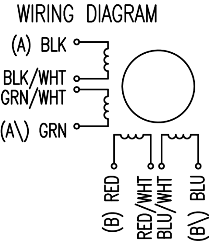
Рис. 3.10: Контакты мотора
