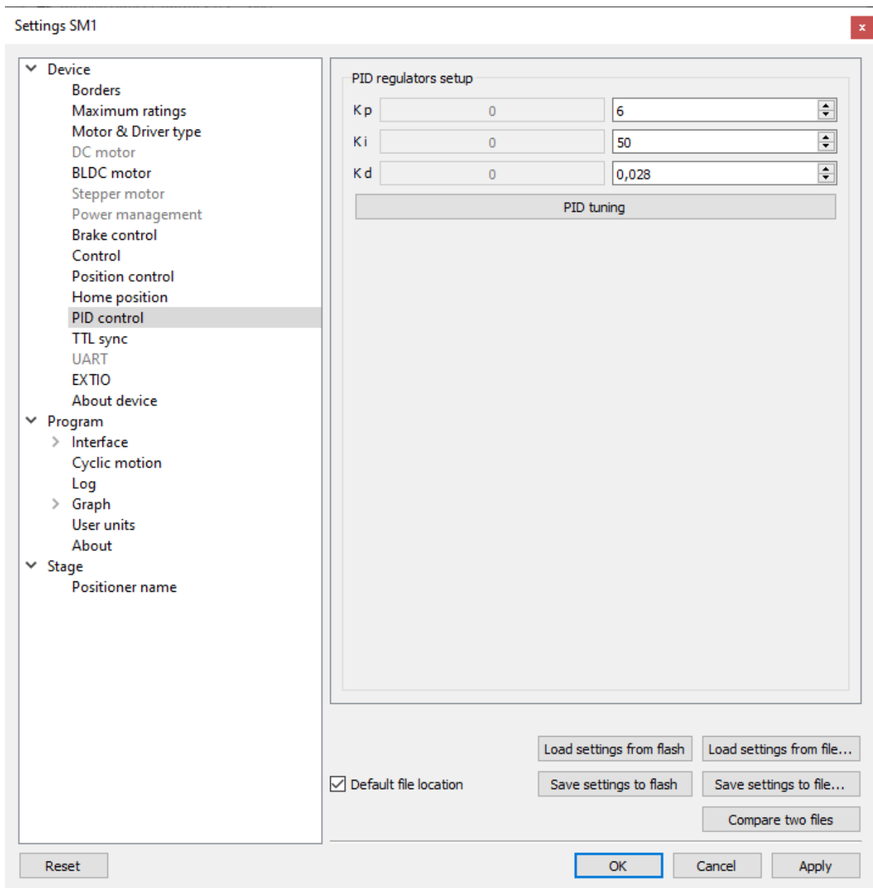
Рис. 5.31: Окно настройки контуров PID-регулирования
