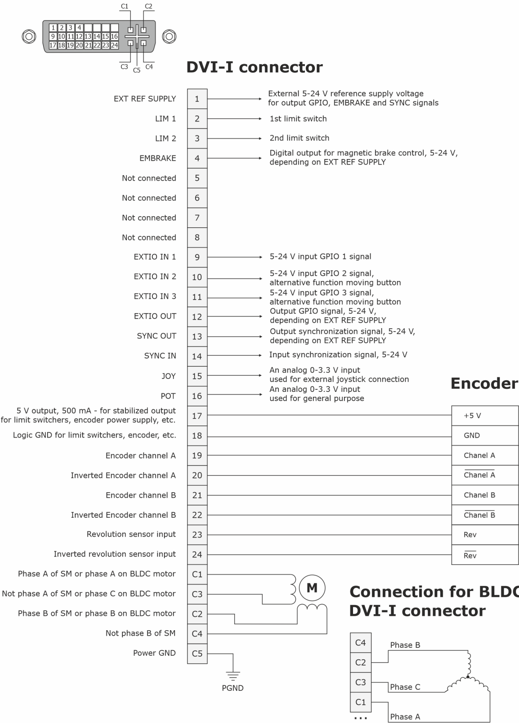
Рис. 3.7: Общая схема подключения позиционера с энкодером через разъем DVI-I
