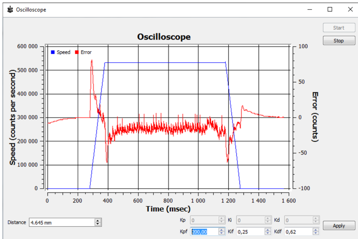
Рис. 4.16: Окно настройки PID-регулятора.
