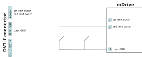
Рис. 4.18: Подключение концевиков типа «сухой контакт»
