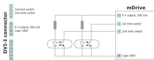
Рис. 4.17: Подключение концевиков типа «оптопара»
