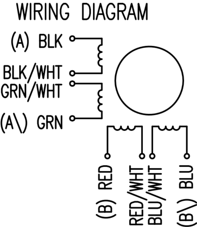
Рис. 3.10: Контакты мотора
