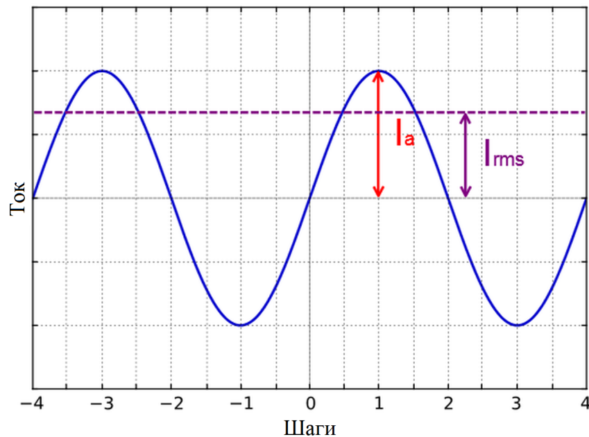
Рис. 3.26: Оциллограмма тока обмотки двигателя и расчёт среднеквадратичного значения
