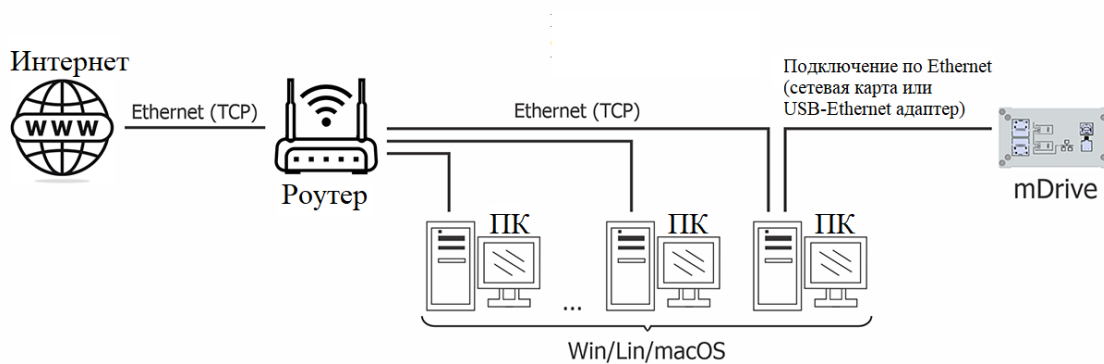
Рис. 7.4: Прямое подключение контроллера mDrive к ПК, подключенному к локальной сети с выходом в сеть Интернет, доступ к управлению ограничен данным ПК
