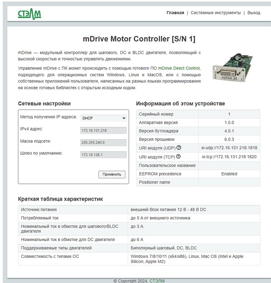
Рис. 8.9: Веб-панель mDrive
