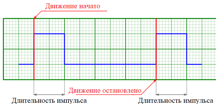
Рис. 4.41: Выходные импульсы синхронизации при генерации их на старте и на остановке движения (импульс фиксированной длительности)
