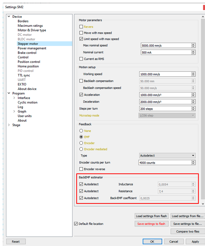
Рис. 4.19: Настройки BackEMF-estimator
