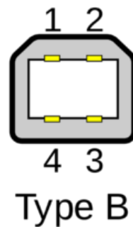
Рис. 4.8: Разъем USB type-B
