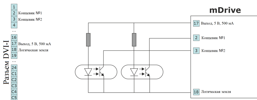
Рис. 4.21: Подключение концевых выключателей типа «оптопара»
