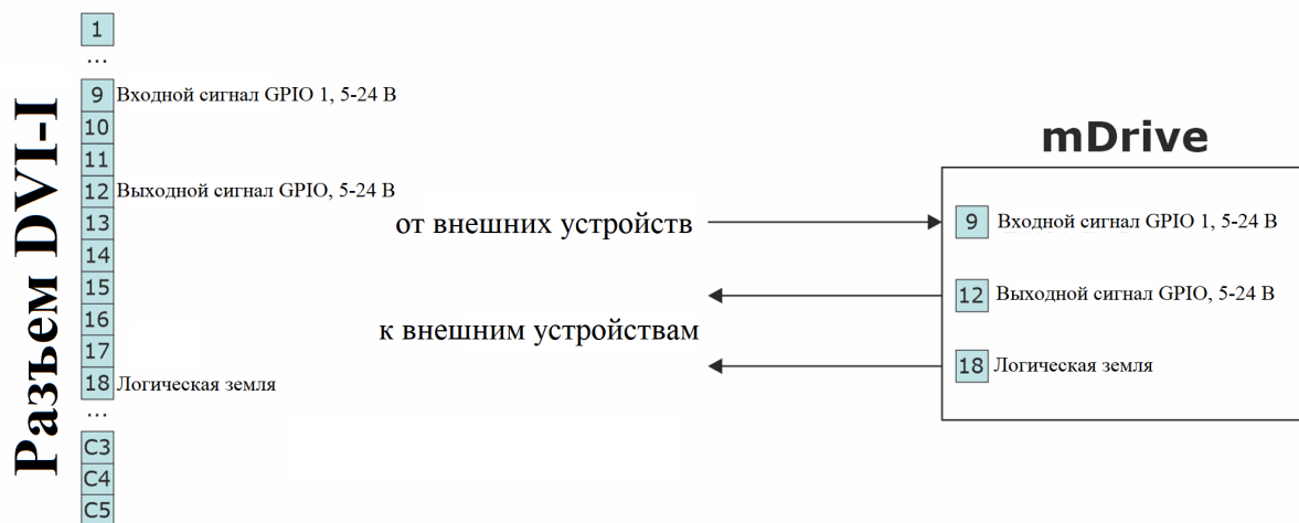
Рис. 4.48: Схема подключения к цифровому входу и выходу на плате контроллера
