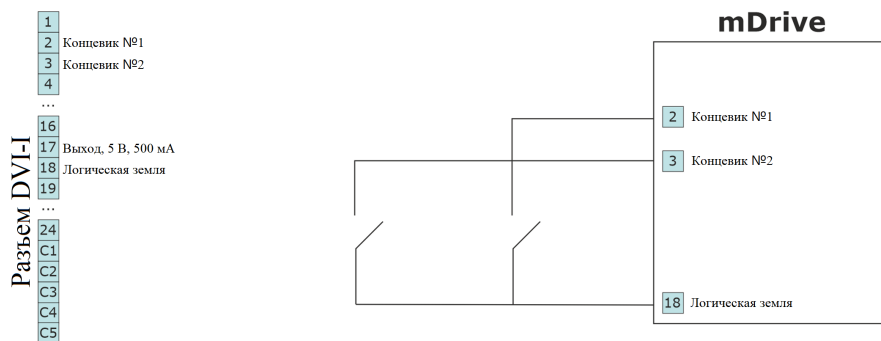
Рис. 4.22: Подключение концевых выключателей типа «сухой контакт»
