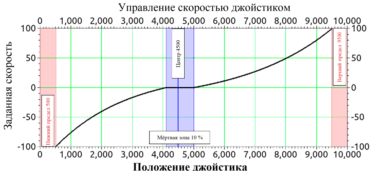
Рис. 4.32: Пример зависимости скорости движения от отклонения джойстика
